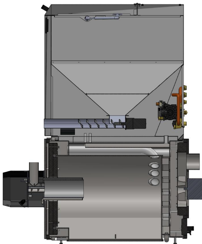
Obrázek 2 Řez kotle
