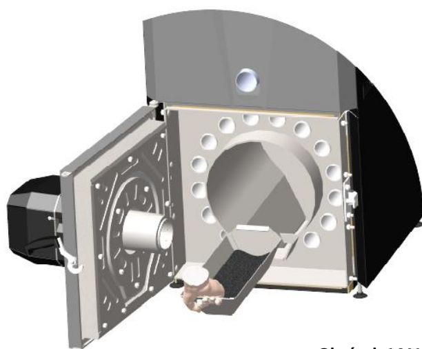
Obrázek 14 Vytažení popelníku z kotle
