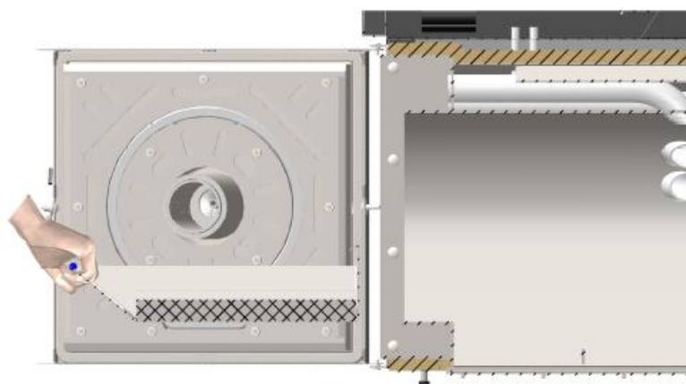
Obrázek 14 Vytažení popelníku z kotle
