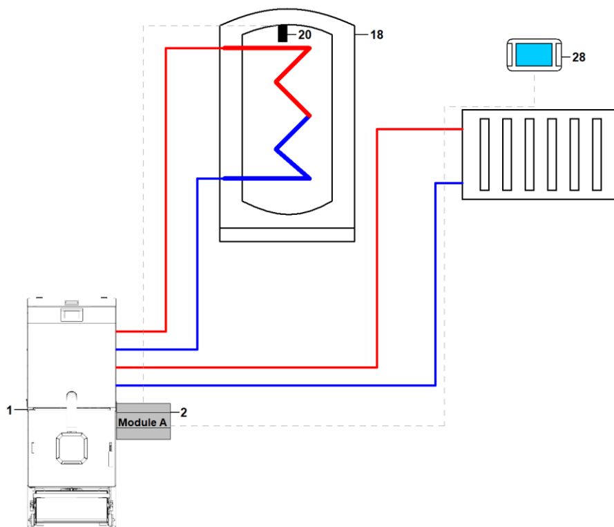
1 – kotel RP Compact, 2- regulátor, 18 – zásobník TUV, 20 – čidlo teploty TUV, 28 – ecoSTER
